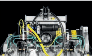
喷水系统（标准和高流量）能够有效冷却刀齿，从而延长刀齿的使用寿命
